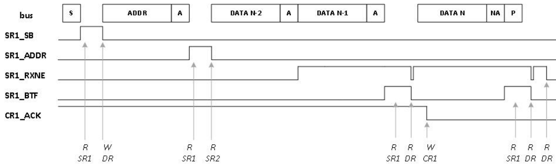
图12- 5 主接收模式（非及时、3 字节）示意图
