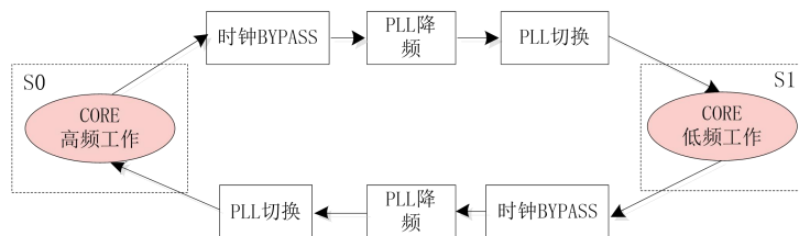
图26- 1 处理器核 DFS 操作流程图
