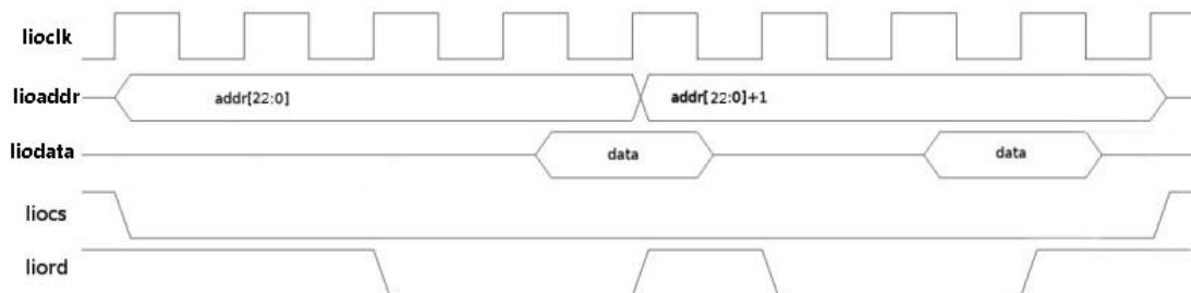
图13- 1 LocalIO 读时序
