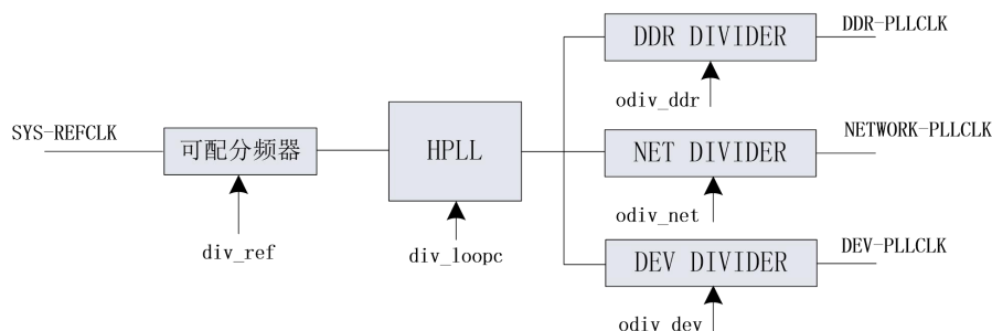
图2- 3 DDR PLL 时钟结构
