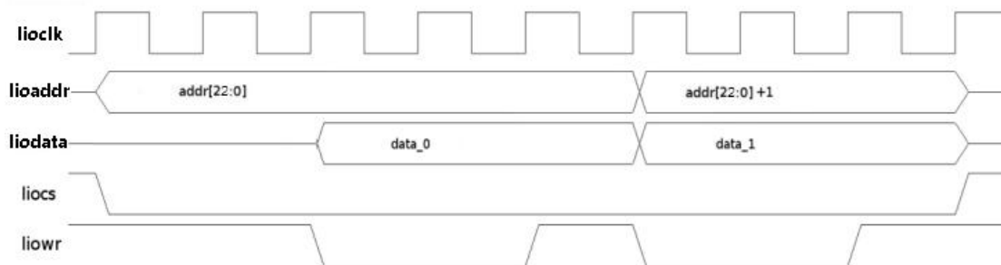
图13- 2 LocalIO 写时序
