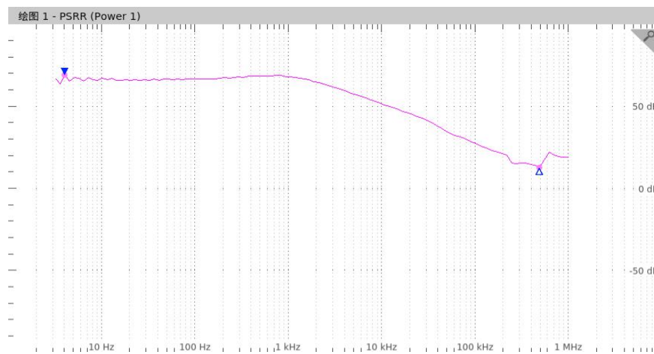
PSRR 曲线
