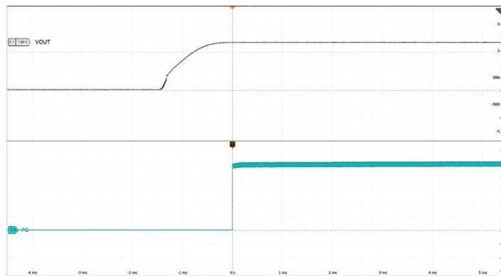
软启动波形
