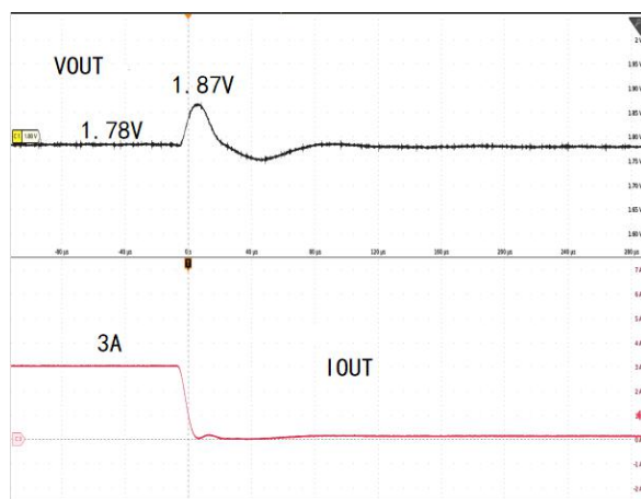
VOUT=1.8V 的 3A 负载跳变瞬态波形
