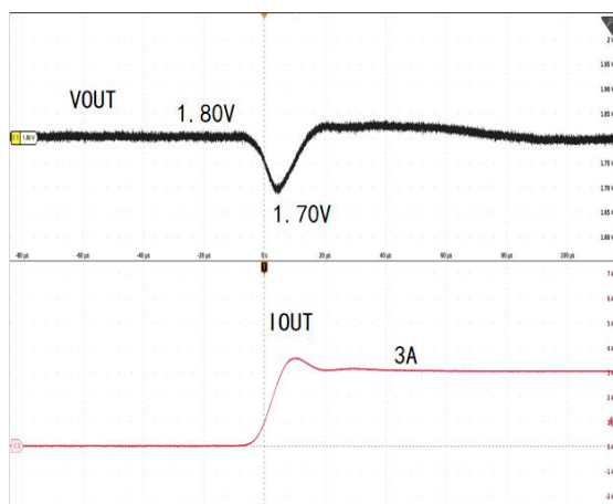
VOUT=1.8V 的 3A 负载跳变瞬态波形
