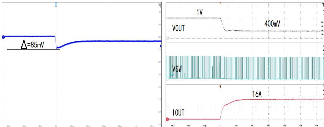
负载跳变 (0A~10A)
