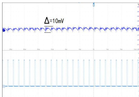
空载的稳态工作波形
