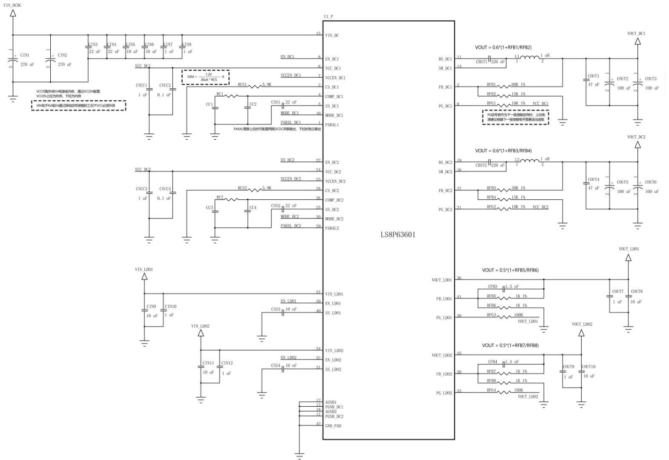
图 4 LS8P63601 典型应用
