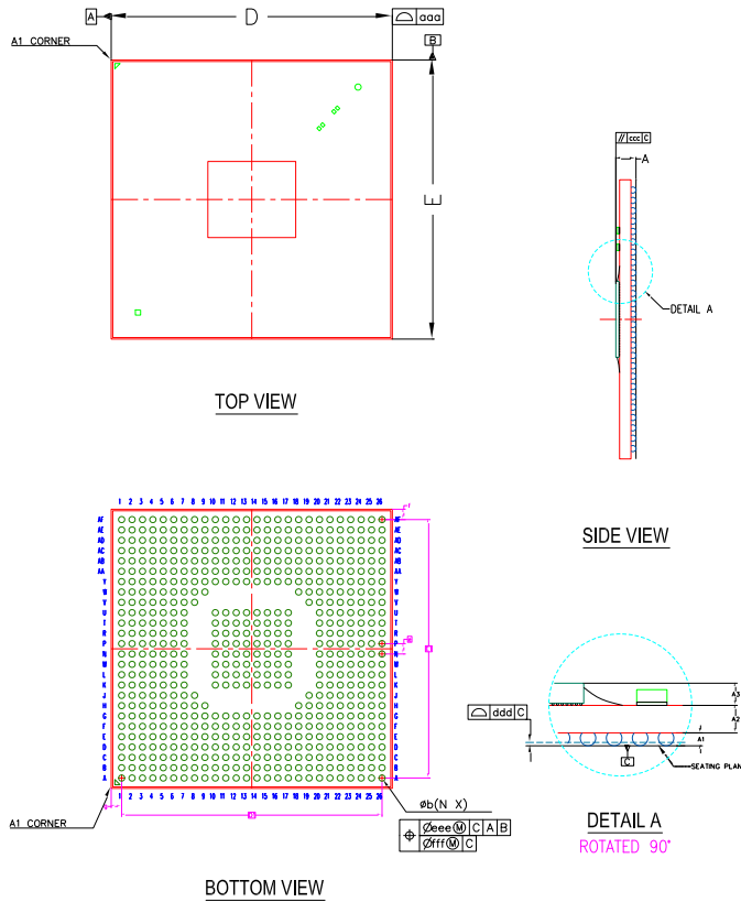
图 7-2 B 版封装尺寸
