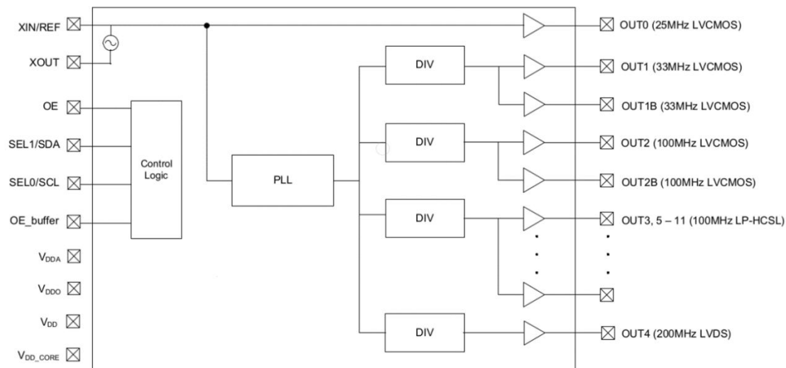
图 3 功能框图
