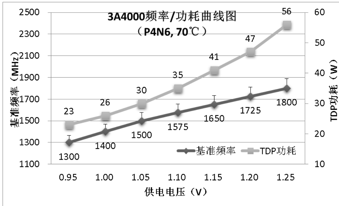
图 7.1 P4N6 偏压和 70 度亮温，基准频率和TDP曲线
