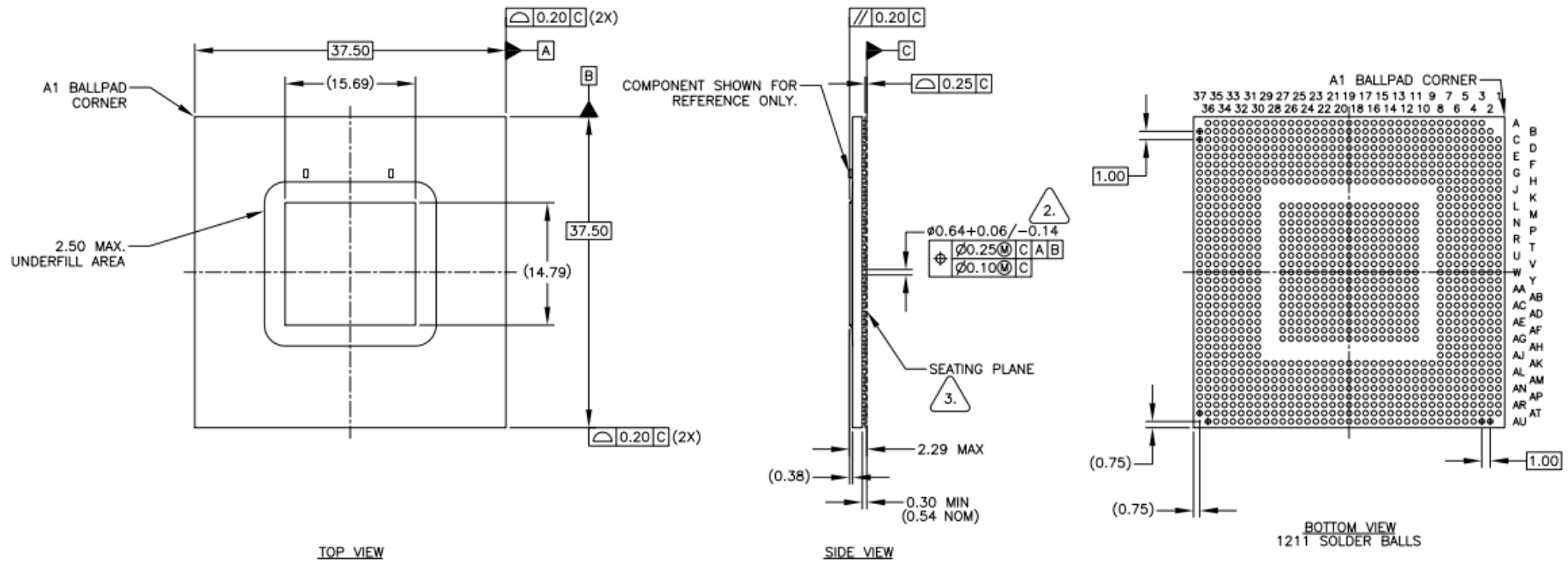
图 11.2 龙芯 3A4000M 顶视图、侧视图和底视图
